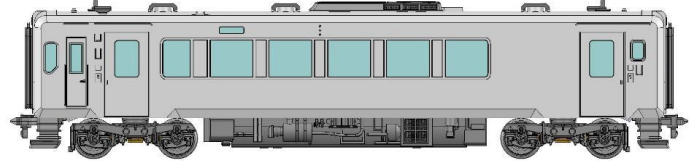
運転室窓は2次車同様のHゴム窓
