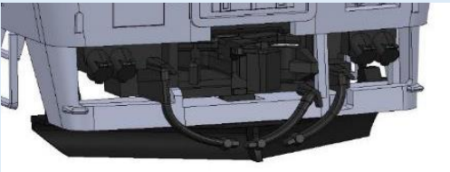
キハ40-1801形2エンド側のスカート ※ジャンパホースの取付は不可となります
