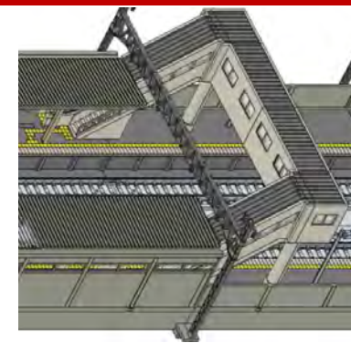
対向式ホーム端部への設置例
