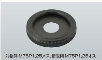
対物側:M75P1.25メス、接眼側:M75P1.25オス
