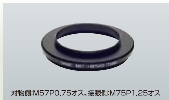
対物側:M57P0.75オス、接眼側:M75P1.25オス
