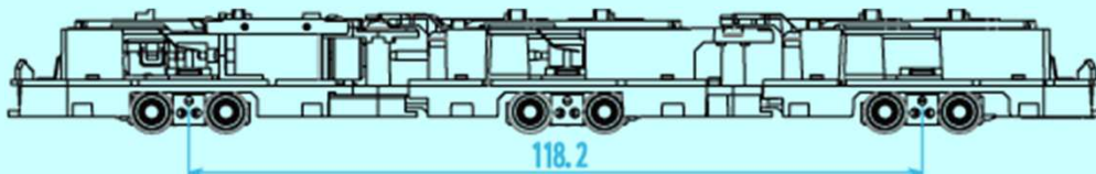
F1000形“FUKURAM”専用動力ユニットTM-LRT04 LRT用3連接発売！
